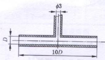
b) 燃气测压管
