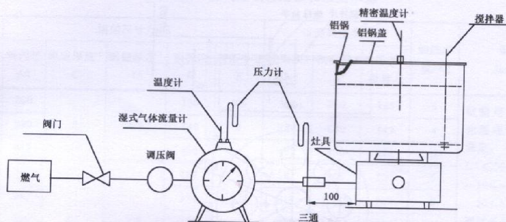
a) 试验装置连接图
