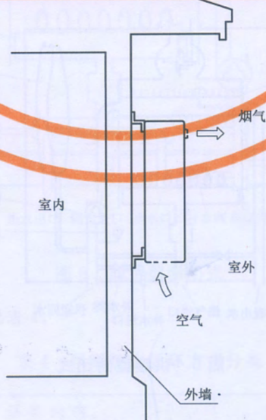
图4 室外型
