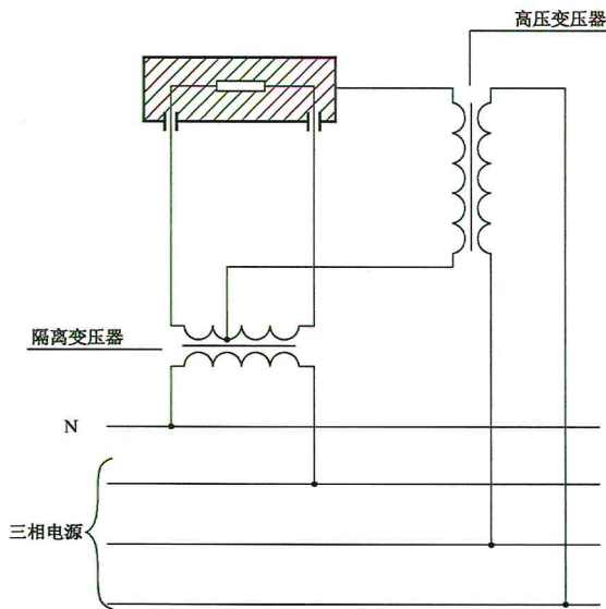
图 14 测量泄漏电流的电路图
