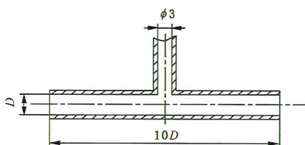
b) 燃气测压管
