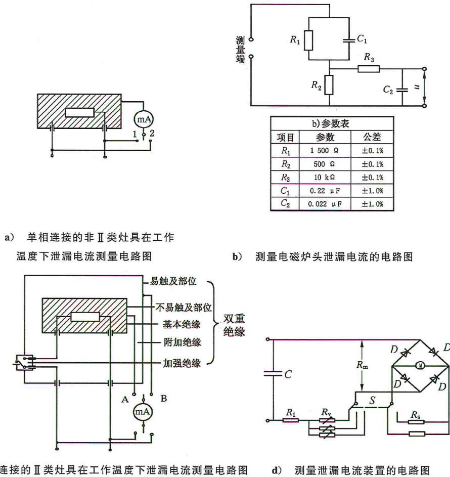
图 14 测量泄漏电流的电路图
