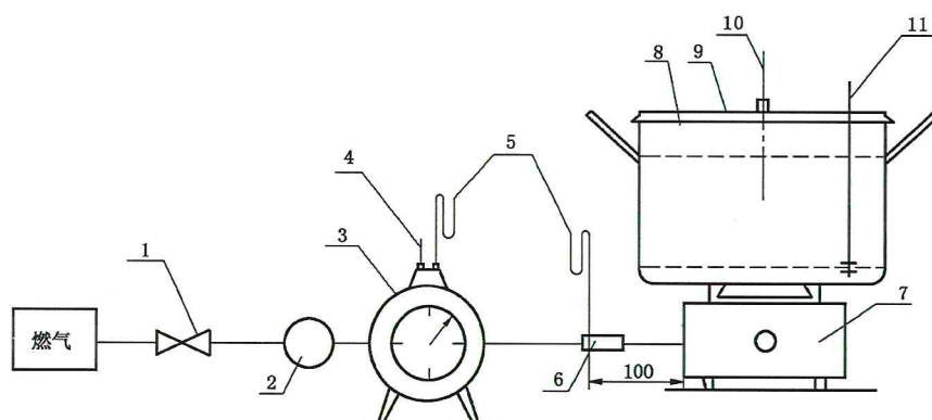
a) 试验装置连接图
