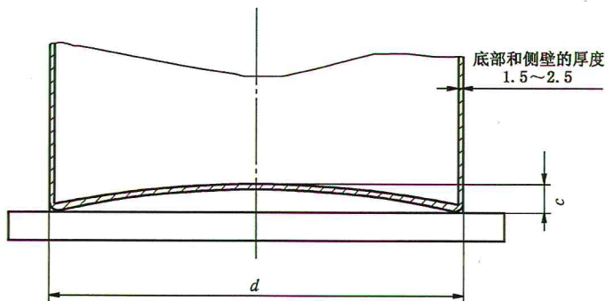
图 7 电灶头试验用锅
