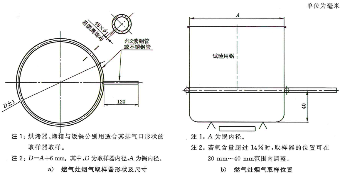
图 6 烟气取样器及取样位置
