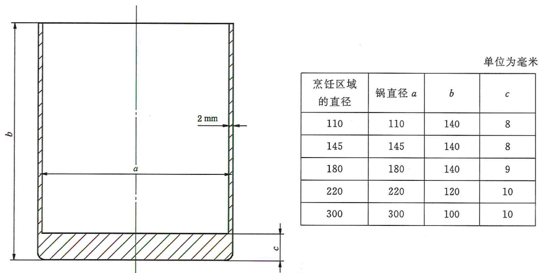
图 7 电灶头试验用锅
