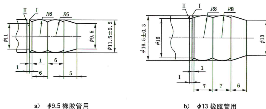
a) \phi 9.5 橡胶管用
