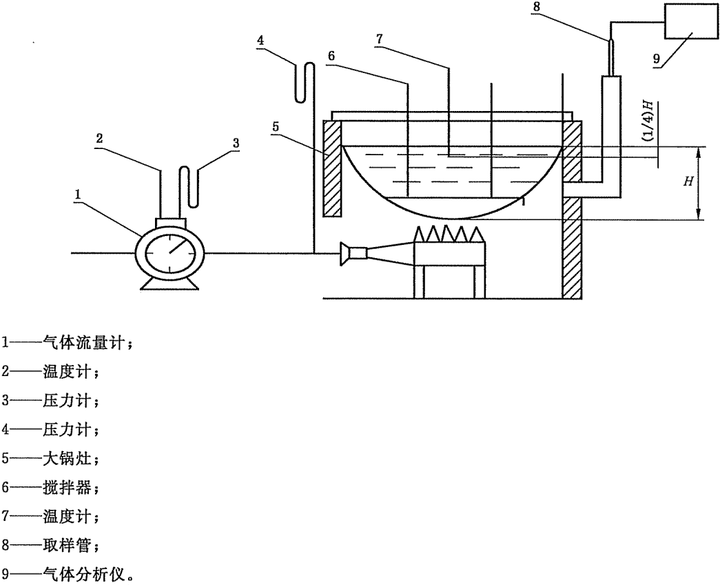
图 1 试验系统
