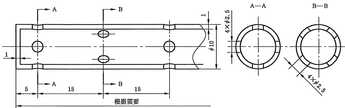
图2 取样管
