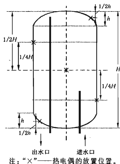
图2 立式安装的热电偶放置
